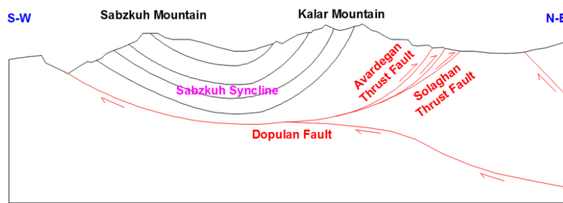
شکل ۴. اجزای زمین‌ریخت - ساختاری محدوده مورد مطالعه
