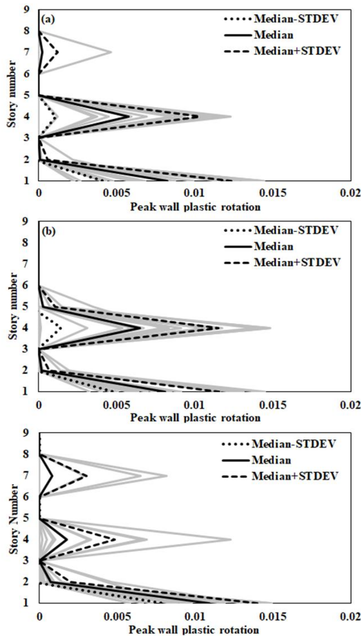
شکل ۱۱. نمودار حداکثر دوران پلاستیک دیوارهای ساختمان نه طبقه در طبقات مختلف و در سطح شتاب طیفی فروریزش با
