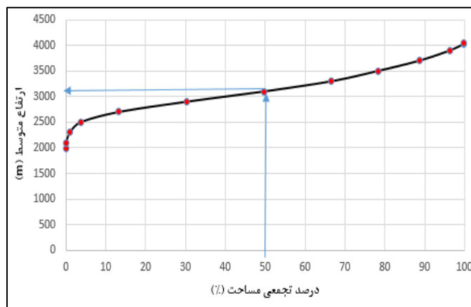
شکل ۸-الف: نمودار هیپسومتری حوضه آبرگیر چشمه کارستی ورسخوران Fig. 8. Hypsometric diagram of Vorsakhuran karst spring catchment basin
