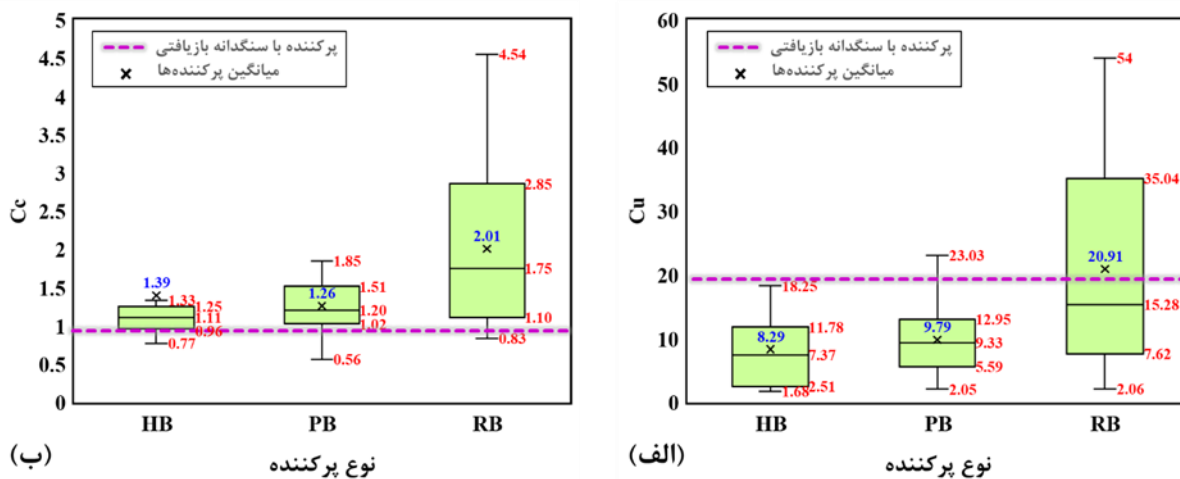
شکل ۲۰. نمودار جعبه‌ای مربوط به (الف) ضریب یکنواختی و (ب) ضریب انحناهای پرکننده‌های هیدرولیکی، خمیری و سنگی به همراه پرکننده حاصل از سنگدانه بازیافتی
