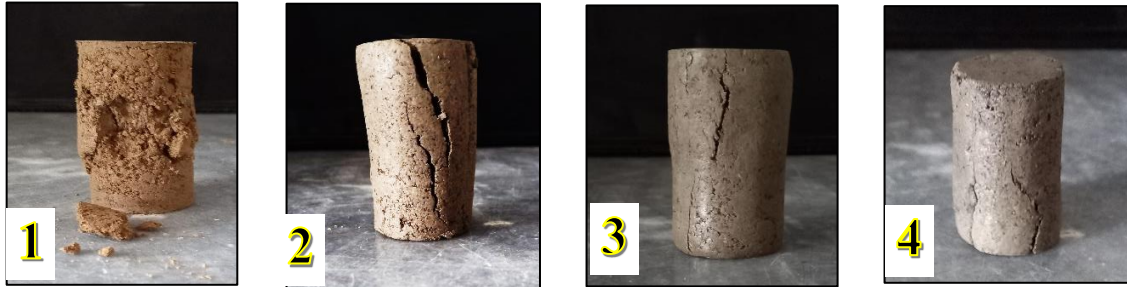
شکل ۷. نحوه شکست نمونه‌های خاک بدون افزودنی و مسلح شده با خاکستر پوسته برنج
