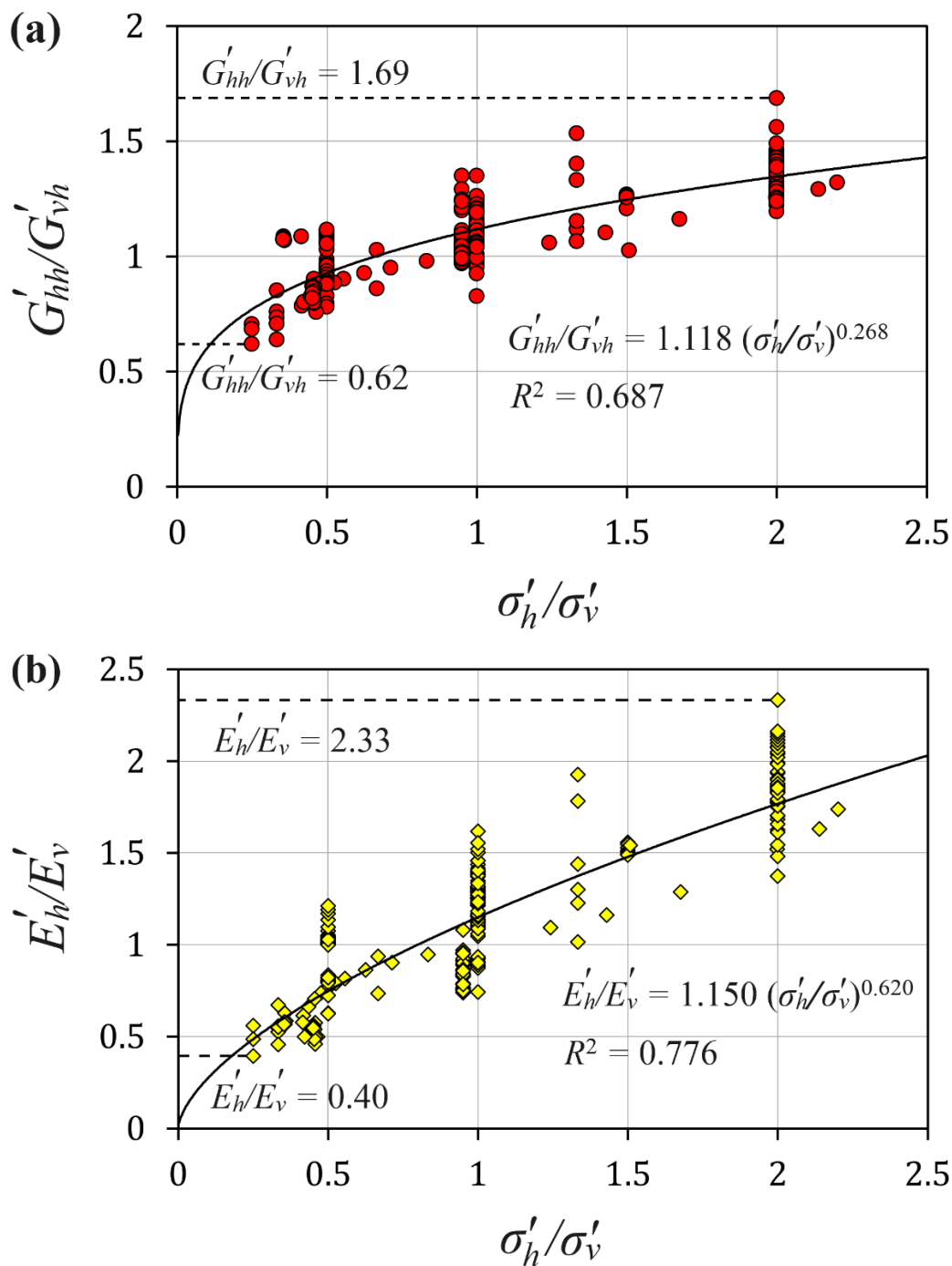
شکل ۱. مدل تغییرات نسبت‌های ناهمسانگردی (a) مدول برشی G'_{hh}/G'_{vh} و (b) مدول یانگ E'_h/E'_v در برابر نسبت تنش \sigma'_h/\sigma'_v در خاک‌های غیر چسبنده
