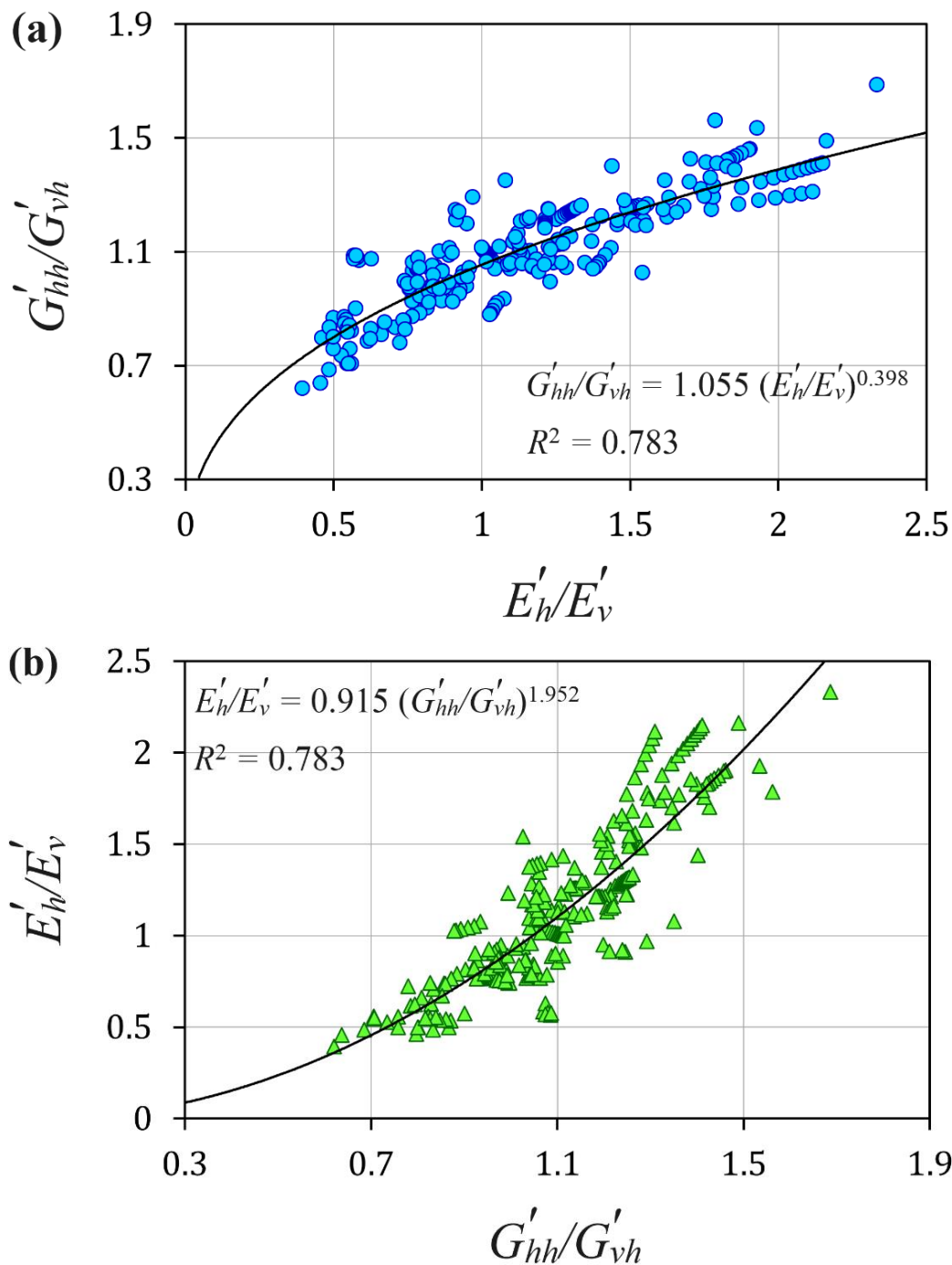
شکل ۲. ترسیم متقابل نسبت‌های ناهمسانگردی مدول برشی و مدول ینگ در برابر یکدیگر و ارزیابی همبستگی بین آن‌ها. (a) نمایش G'_{hh}/G'_{vh} به صورت تابعی از E'_h/E'_v ; (b) نمایش E'_h/E'_v به صورت تابعی از G'_{hh}/G'_{vh}
