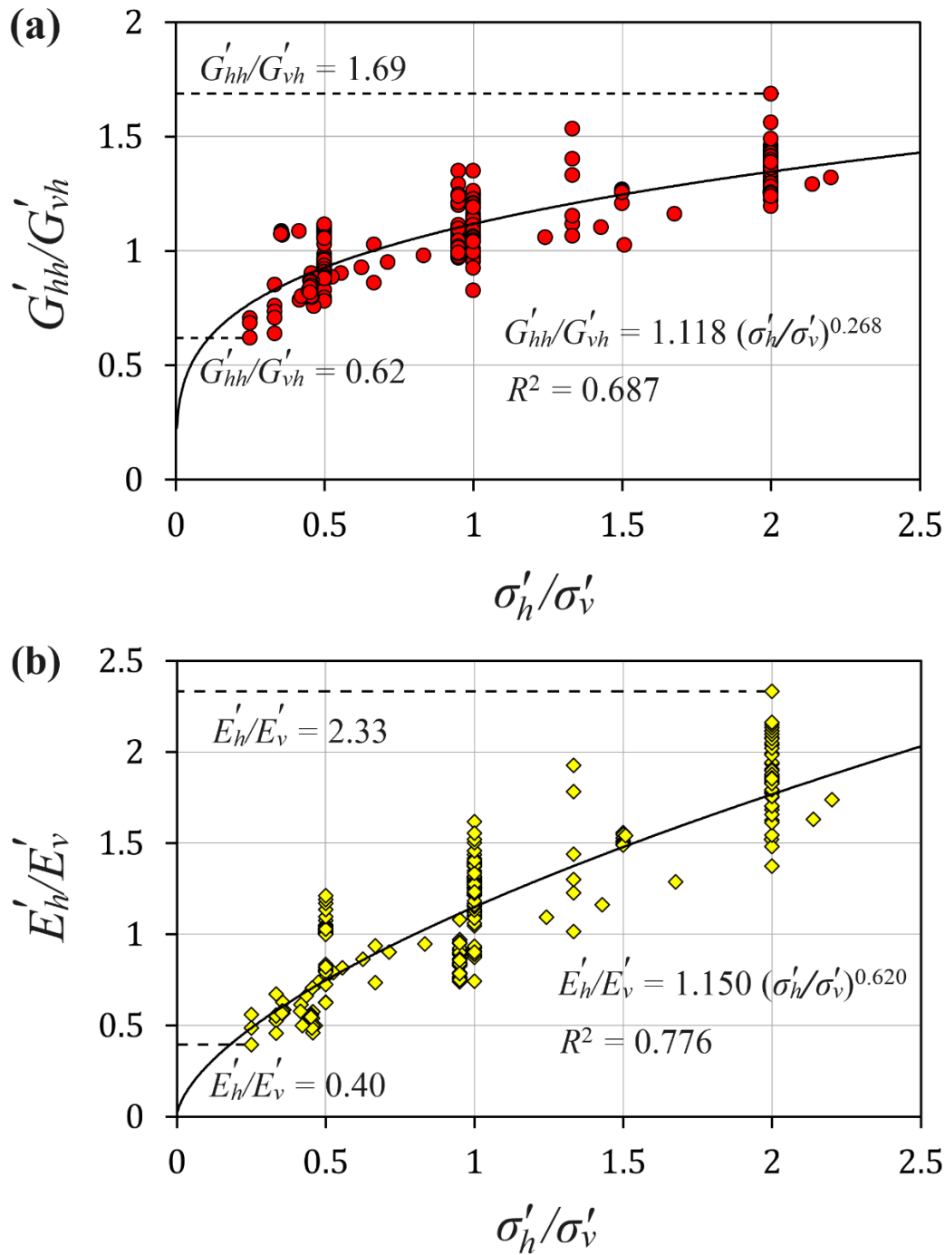
شکل ۱. مدل تغییرات نسبت‌های ناهمسانگردی مدول برشی G'_{hh}/G'_{vh} و (a) مدول برشی G'_{hh}/G'_{vh} و (b) مدول یانگ E'_h/E'_v در برابر نسبت تنش \sigma'_h/\sigma'_v در خاک‌های غیر چسبنده
