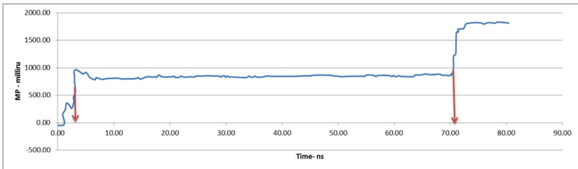
شکل 5. موج TDR برای کابل دو رشته‌ای مخابراتی و تعیین ابتدا و انتهای کابل. Fig. 5. TDR wave for Bi-wire telecommunication cable and determining the beginning and end of the cable.
