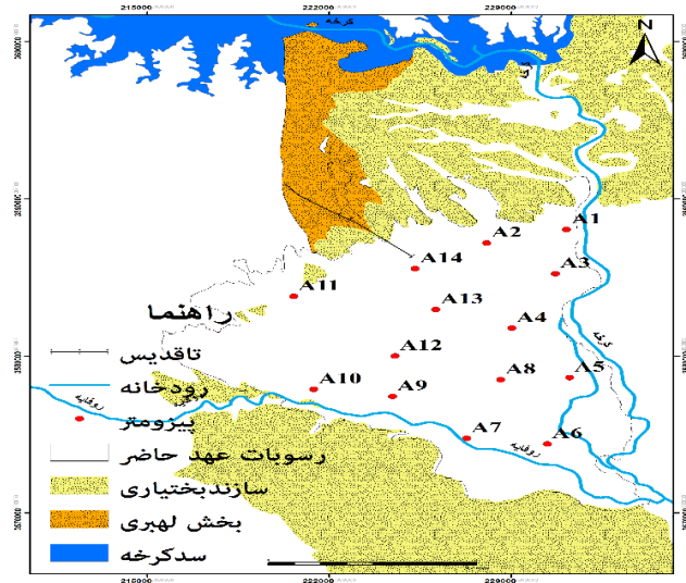
شکل ۱. موقعیت جغرافیایی و محل چاه‌های مشاهداتی دشت اوان Fig. 1. Geographical location and location of observation wells in Evan plain
