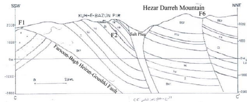
۱۲- ج - برش زمین شناسی CC-CC
