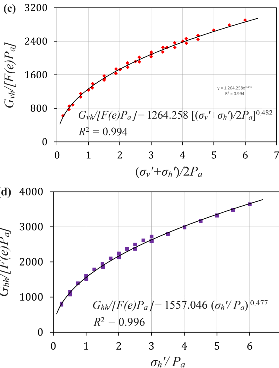
شکل ۷. فرآیند به‌دست آوردن ثابت‌های A_{vh} و A_{hh} برای ماسه کنیا در حالت‌های نسبتاً شل و متراکم. (a) ترسیم G_{vh}/F(e)P_a در برابر (\sigma'_v + \sigma'_h)/2P_a به منظور استخراج A_{vh} برای نمونه‌هایی با D_r = 30-40\% ; (b) ترسیم G_{hh}/F(e)P_a در برابر \sigma'_h/P_a به منظور استخراج A_{hh} برای نمونه‌هایی با D_r = 30-40\% ; (c) ترسیم G_{vh}/F(e)P_a در برابر (\sigma'_v + \sigma'_h)/2P_a به منظور استخراج A_{vh} برای نمونه‌هایی با D_r = 85-95\% ; (d) ترسیم G_{hh}/F(e)P_a در برابر \sigma'_h/P_a به منظور استخراج A_{hh} برای نمونه‌هایی با D_r = 85-95\% .
