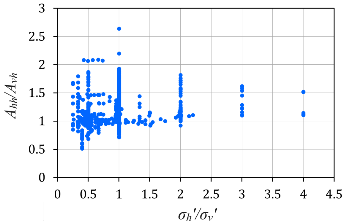
شکل ۴. ترسیم تغییرات A_{hh}/A_{vh} در مقابل نسبت تنش \sigma'_h/\sigma'_v در خاک‌های دانه‌ای ( N = 1042 )
