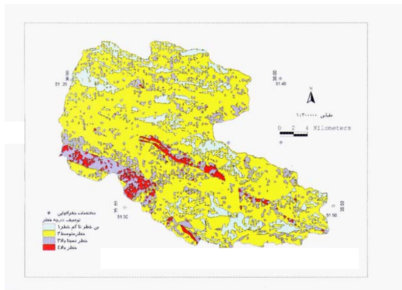
شکل ۸: نقشه پهنه‌بندی خطر زمین لغزش حوزه آبخیز سد لتیان به روش تراکم سطح
