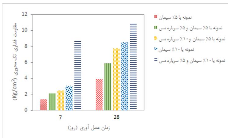
شکل ۱۵-تاثیر زمان عمل‌آوری بر مقاومت فشاری تک‌محوری نمونه‌های ساخته‌شده با تراکم ۹۵ درصد و رطوبت سمت
