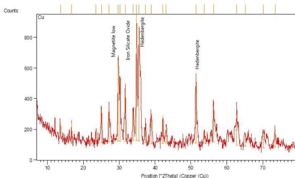
شکل ۶- آنالیز XRD نمونه سرباره
