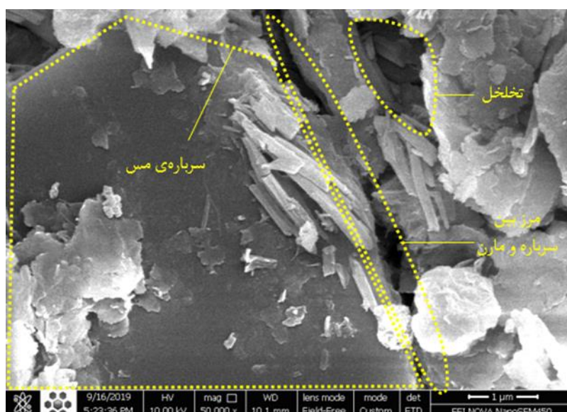
شکل ۲۳- خاک مارن مورد مطالعه تثبیت‌شده با ۱۰ درصد سیمان و پنج درصد سرباره‌ی مس
