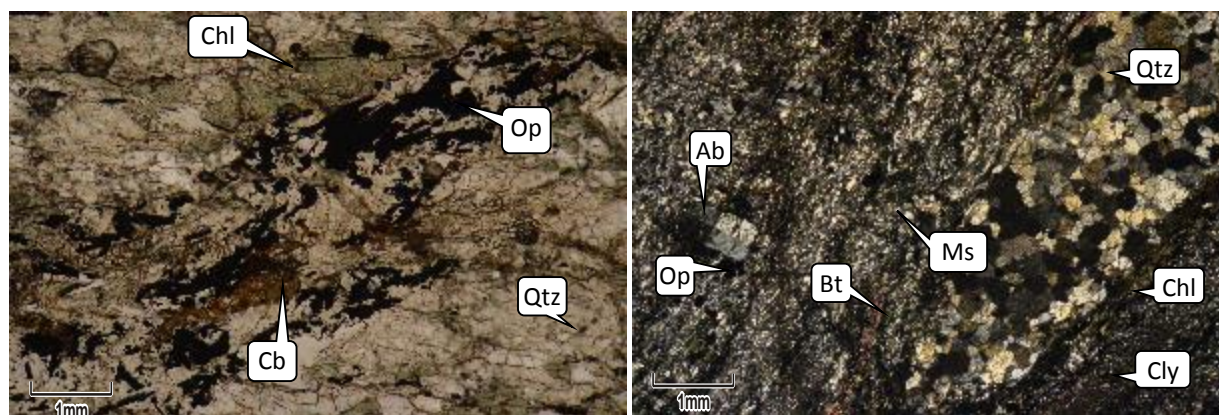
شکل شماره-۶، مقطع کانی‌شناسی شیست (C2) - بخش عمده نمونه از کانی کوارتز با لایه‌بندی ریز و درشت مشاهده می‌شود (نور عبوری XPL). (سمت راست)؛ کلریتی شدن، کربناتی شدن و نفوذ سیال کانه زا در امتداد شیستوزیته مشاهده می‌شود (نور عبوری PPL). (سمت چپ).
