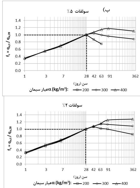
شکل ۱۰. تغییرات مقدار پارامتر f_c در سنین مختلف به ازای عیارهای مختلف سیمان (200, 300, 400 \text{ kg/m}^3) (در سولفات الف) ۵٪ و ب) ۲٪.
