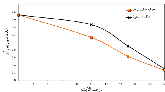
شکل ۱۲. اعداد سی بی آر برای درصد‌های گوناگون دو ماده آلاینده گلیسرول و استون
