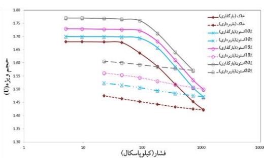
شکل ۸. نتایج آزمایش تحکیم شامل تغییرات حجم ویژه با بار اعمال شده در حین بارگذاری و باربرداری برای خاک طبیعی و خاک اختلاط یافته با استون
