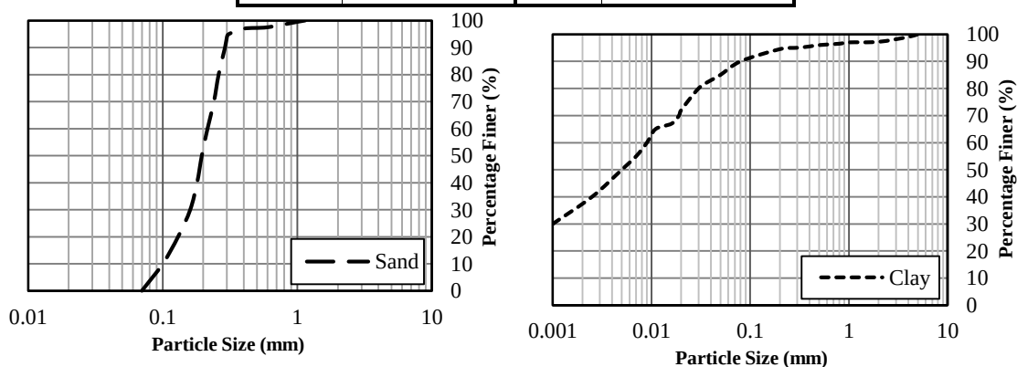
شکل ۱. توزیع دانه‌بندی ماسه و رس.
