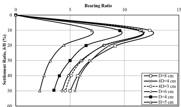
شکل ۱۳. تغییرات نسبت ظرفیت باربری-نسبت نشست نمونه‌های رس + تک/گروه ستون‌های ماسه‌ای + ماسه سطحی غیرمسلح.
