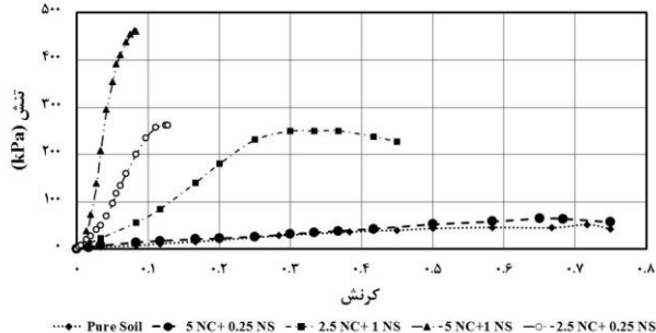
شکل ۱۱. بررسی پارامتر مقاومت فشاری در نمونه‌های بهسازی شده با مقادیر متفاوت هیبرید نانوذرات
