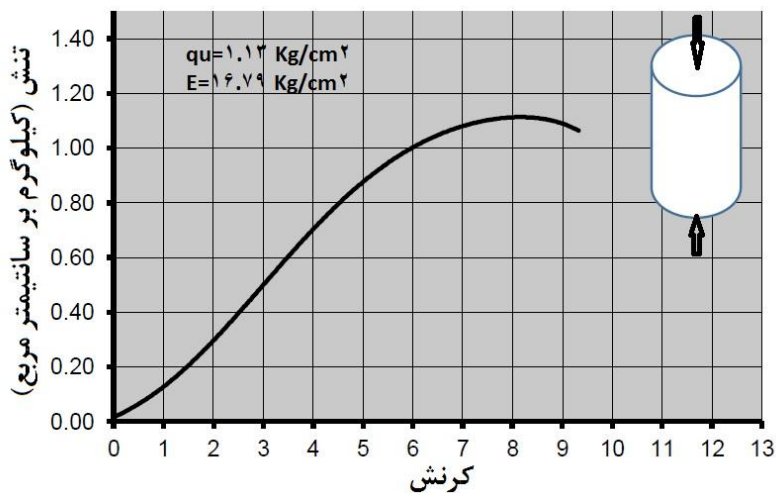
شکل ۵. نمودار تنش-کرنش در آزمایش مقاومت فشاری تک محوری برای نمونه خاک با ۰/۵ درصد نانوکائولینیت
