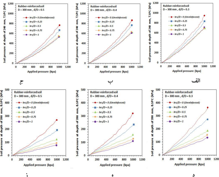
شکل ۱۲. نمودار تغییرات تنش اندازه‌گیری شده به وسیله فشارسنج‌های الف، ب، ج) فوقانی (T.SPC) در عمق ۲۴۰ میلی‌متر د، ه، ز) تحتانی (B.SPC) در عمق ۳۹۰ میلی‌متر، در برابر فشار اعمالی بر پی‌های رینگى با نسبت قطر داخلی به خارجی مختلف (۰/۳، ۰/۴، ۰/۵) و مستقر بر بستر مسلح شده با لایه خاک-خرده لاستیک با ضخامت‌های متغیر
