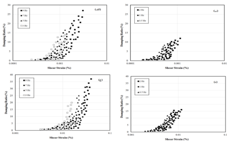
شکل ۲۲. تغییرات نسبت میرایی با کرنش برشی در فرکانس‌های مختلف بارگذاری تحت بارگذاری سینوسی و شتاب ورودی الف و ب (۰/۱g، ج و د) ۰/۳g
