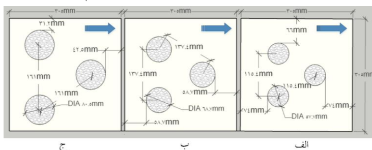
شکل ۱۰. آرایش قرارگیری ستون‌های سنگی در آرایش مربعی الف (۸/۴، ب) ۱۲/۴، ج) ۱۶/۴، د) نمونه ساخته شده در دستگاه برش مستقیم
