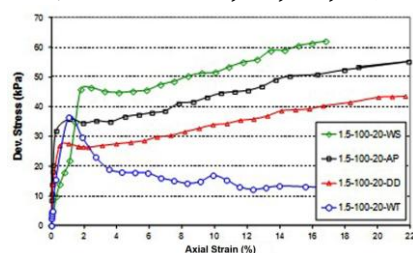
شکل ۹. نمودارهای مسیر تنش ترکیبات ماسه و رس
