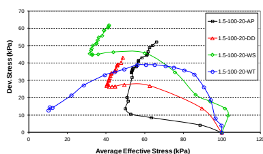
شکل ۷. نمودارهای مسیر تنش ترکیبات ماسه و رس
