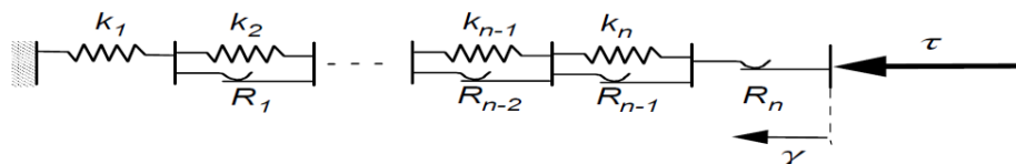
شکل ۵. نمایش شماتیک مدل تنش-کرنش استفاده شده
