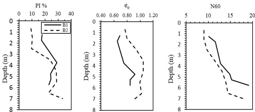
شکل ۶. نمودار تغییرات متغیرهای مهم تحقیق نسبت به عمق گمانه‌های حفر شده
