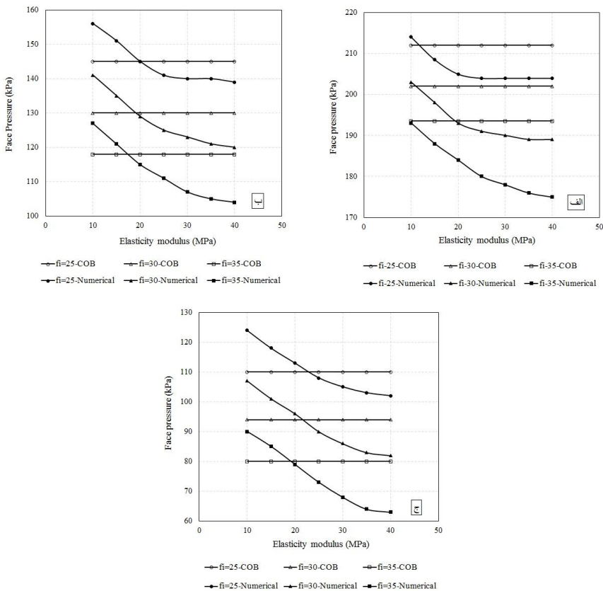
شکل ۷. مدول الاستیسیته - فشار جبهه کار برای تراز آب الف (ب، ج، د)، ج ۲۷ متری از سطح زمین
