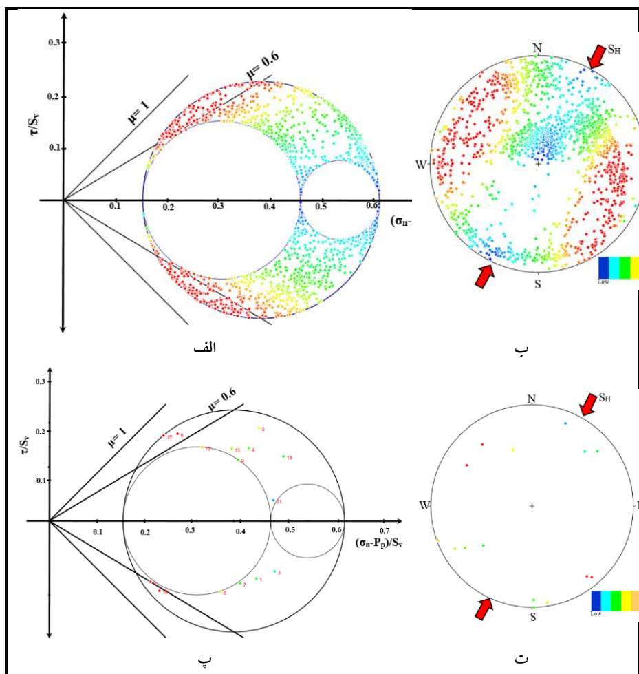
شکل ۱۴. دیاگرام موهر سه‌بعدی برای شکستگی‌ها و گسل‌ها برای پیدا کردن گسل‌ها و شکستگی‌ها بحرانی و تراوا الف و ب) دیاگرام موهر سه‌بعدی برای شکستگی‌ها و گسل‌ها است، ب و ت) استریونتهایی هستند که قطب صفحات شکستگی و گسل را نشان می‌دهند (رنگ‌های گرم نشان‌دهنده پتانسیل زیاد برای فعالیت و رنگ‌های سرد نشان‌دهنده پتانسیل کم برای فعالیت است).
