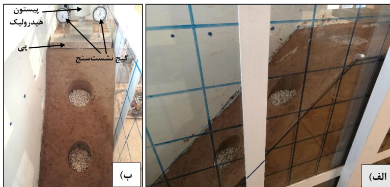
شکل ۱۳. نحوه اجرای گروه سه ستون سنگی غیرمسلح: (الف) سه ستون اجراشده قبل از قرار دادن پی، (ب) ستون‌های اجراشده پس از قرارگیری پی نواری و گيج‌های نشست‌سنج فشار (کیلوپاسکال)
