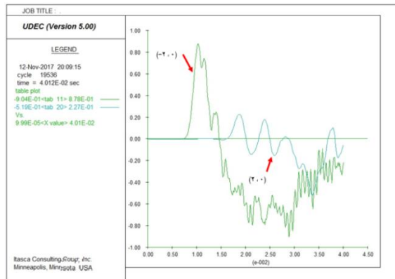
شکل ۱۱. تاریخچهٔ زمانی جابه‌جایی‌های افقی (الف) در نقاط شاهد (0, -2) و (0, 2) روی دیوارهٔ سمت چپ و راست رمپ، (ب) در نقطه شاهد (1/2, 0) روی سقف در مدت زمان ۴۰ میلی ثانیه از اعمال بار دینامیکی
