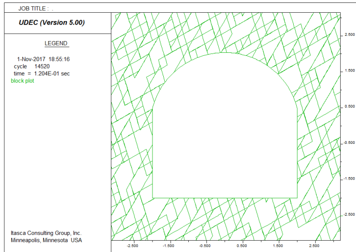
شکل ۶. بزرگ‌نمایی بلوک‌ها پس از تعادل اولیه
