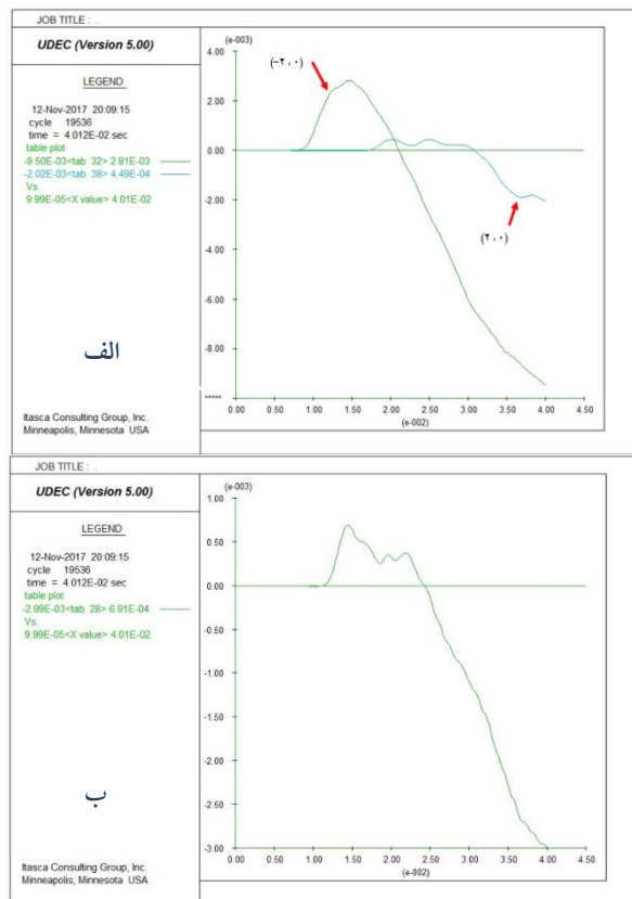
شکل ۱۱. تاریخچه زمانی جابه‌جایی‌های افقی الف) در نقاط شاهد (-۲, ۰) و (۲, ۰) روی دیواره سمت چپ و راست رمپ، ب) در نقطه شاهد (۰, ۲/۱) روی سقف در مدت زمان ۴۰ میلی ثانیه از اعمال بار دینامیکی
