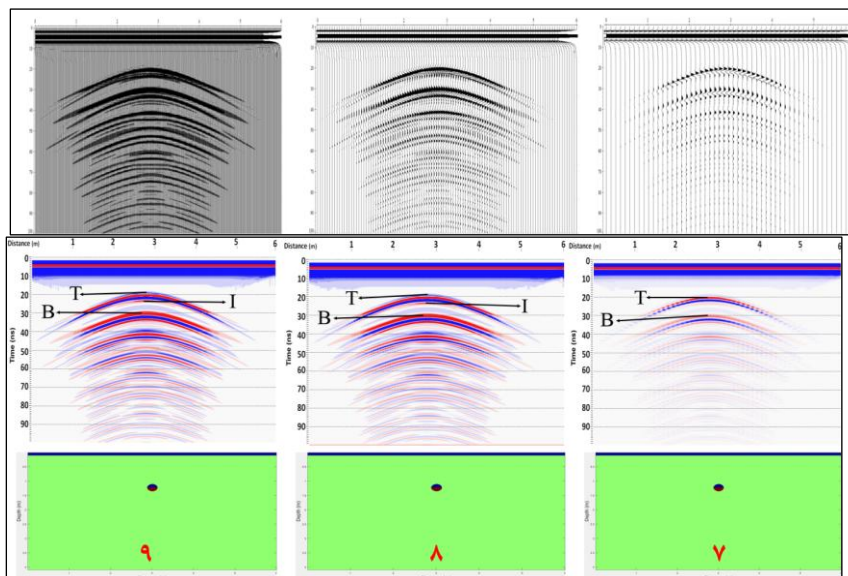
شکل ۵. بررسی تأثیر فاصله نمونه‌برداری مکانی بر پاسخ GPR اهداف استوانه‌ای افقی شامل دو نوع سیال در محیط میزبان از جنس خاک رس سیلتی؛ فاصله نمونه‌برداری مکانی در مدل ۷ برابر با ۱۰ سانتی‌متر و در مدل‌های ۸ و ۹ به ترتیب برابر با ۵ و ۱ سانتی‌متر است. به ترتیب از بالا به پایین پاسخ مد ترپسی، مد نقطه‌ای و مدل هندسی - فیزیکی
