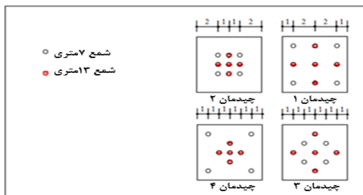
شکل ۶. حالت‌های آرایش پی رادیه-شمع با طول شمع‌های متغیر (واحد: متر)
