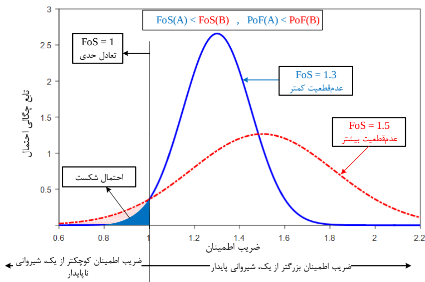
شكل ۱. تأثير عدم قطعیت در توزيع احتمال ضريب اطمینان
