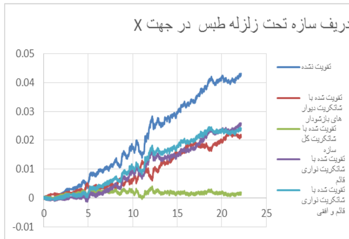
شکل ۱۲. ب) نمودار دریفت سازه تحت زلزله طبس در جهت X
