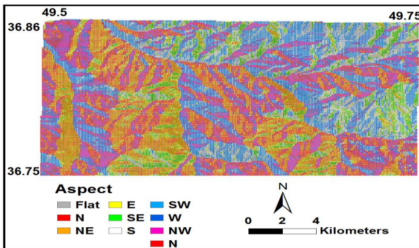
شکل ۸. لایه اطلاعاتی جهت شیب در منطقه بررسی شده
