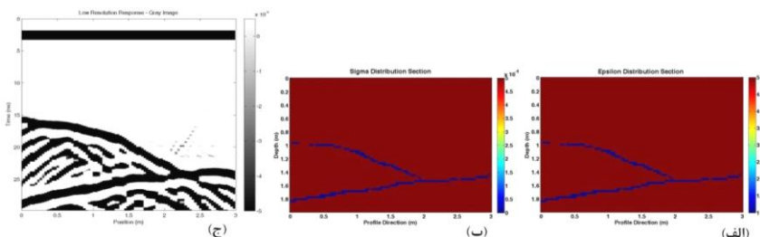
شکل ۶. الف) مقطع توزیع گذردهی دی‌الکتریک، ب) مقطع توزیع هدایت الکتریکی و ج) پاسخ GPR مدل منشور دوبعدی گرانیتی شامل دو ناپیوستگی متقاطع
