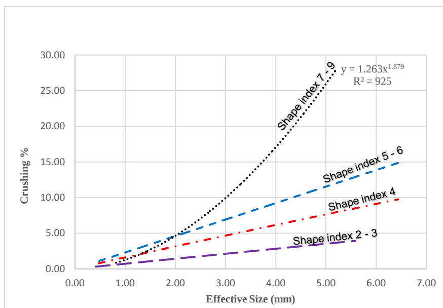
شکل ۱۱. تغییرات خردشده سنگ‌دانه با ضرایب شکل متفاوت
