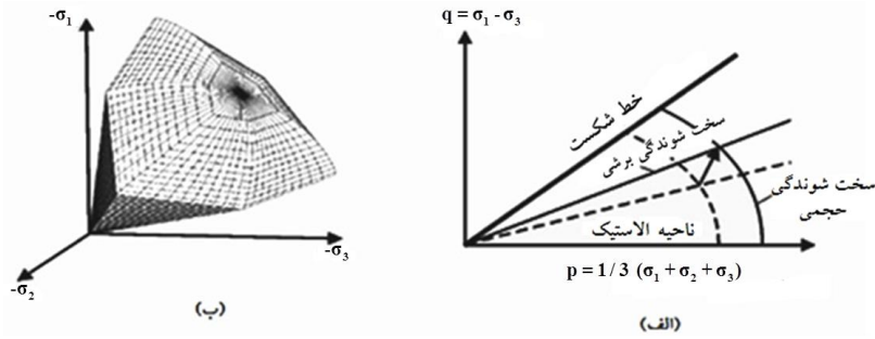
شکل ۶. سطح تسلیم برای مدل خاک سخت شونده در C=0 (الف) سخت شونده گری برشی و حجمی در فضای p-q ، (ب) سطح تسلیم کل در فضای تنش‌های اصلی [۳۱]
