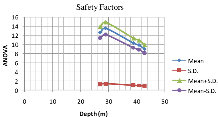
شکل ۸. نمودار آنالیز واریانس برای مقادیر ضریب اطمینان
