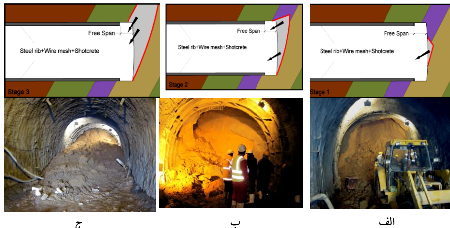
شکل ۴. سازو کار گسیختگی: مرحله اول) گسیختگی موضعی سینه‌کار، مرحله دوم) گسیختگی سقف و کل سینه‌کار، مرحله سوم) گسیختگی دودکش مانند
