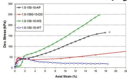
شکل ۶. نمودارهای تنش کرنش محوری ترکیبات ماسه و رس
