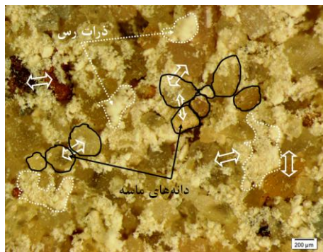
شکل ۱۶. تصویر میکروسکوپی ترکیب ماسه با ۱۰ درصد ریزدانه خمیری با روش DD (بزرگ‌نمایی ۴۰ برابر)
