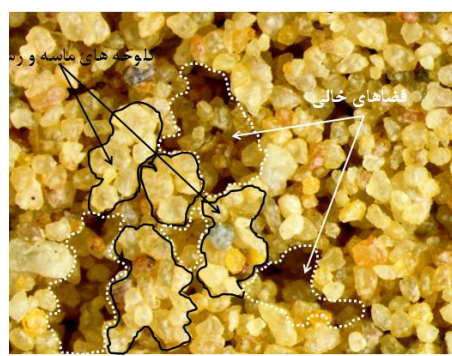
شکل ۱۵. تصویر میکروسکوپی ترکیب ماسه با ۱۰ درصد ریزدانه خمیری با روش WT (بزرگ‌نمایی ۱۶ برابر)
