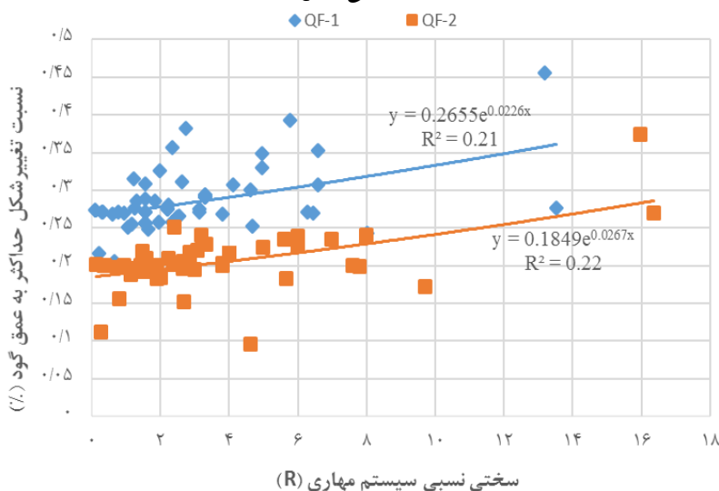
شکل ۱۳. ب) نسبت بیشینه تغییر شکل ایجاد شده به عمق گود در برابر سختی نسبی برای ساختگاه‌های (QF)
