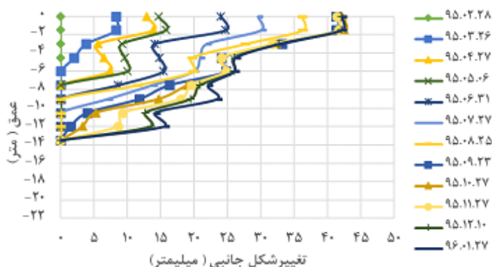
۷. نمودار تغییر شکل جانبی مقطع B در پایش‌های میدانی در تاریخ‌های مختلف
