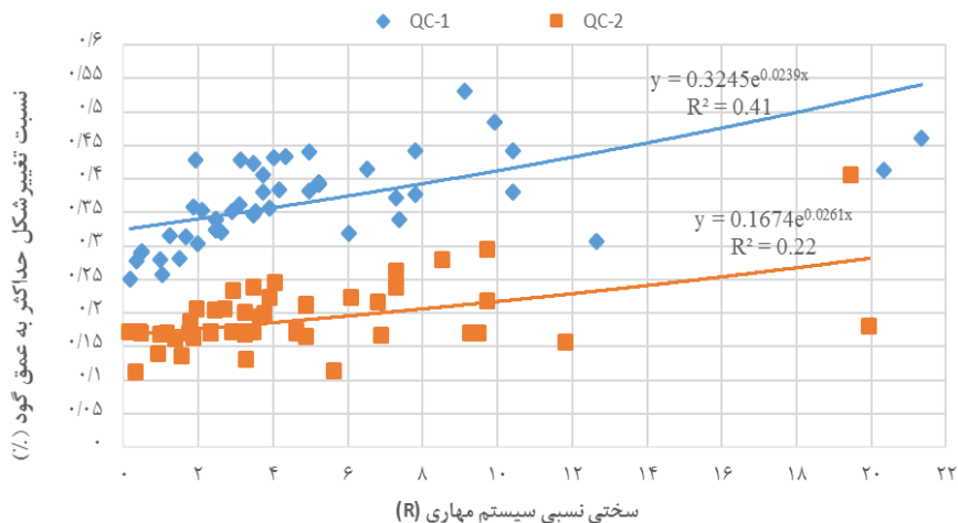
شکل ۱۳. الف) نسبت بیشینه تغییر شکل ایجاد شده به عمق گود در برابر سختی نسبی برای ساختگاه‌های (QC)
