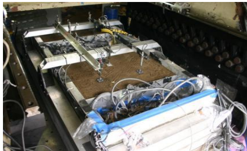
شکل ۴. نمونه‌ای از ابزاربندی یک آزمایش انجام شده در سانتریفیوژ [۱۸]
