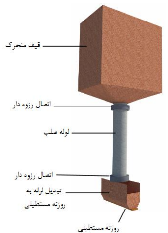
شکل ۳. سیستم انتقال ماسه از قیف متحرک تا روزنه مستطیلی
