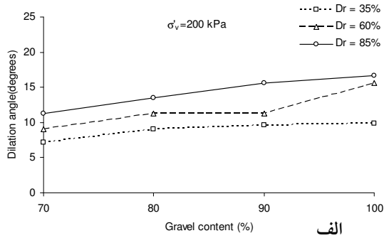
شکل ۲۰. تغییرات زاویه اتساع در مقابل مقدار شن در تراکم‌های نسبی مختلف برای سربارهای مختلف (الف) ۱۰۰ کیلو پاسکال
