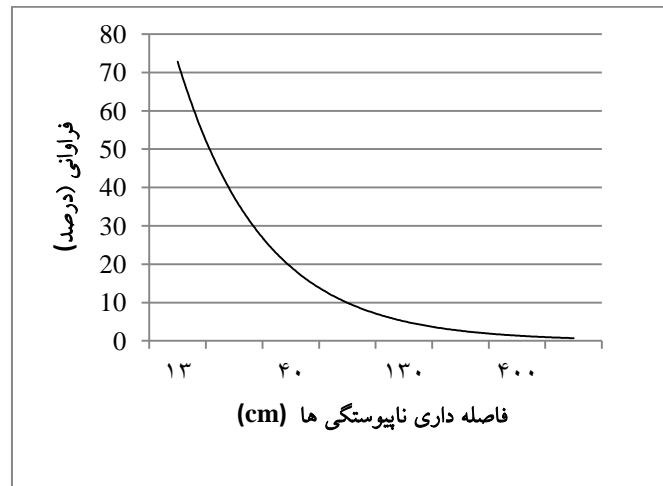
شکل ۳. نمودار فاصله‌داری دسته درزه J1
