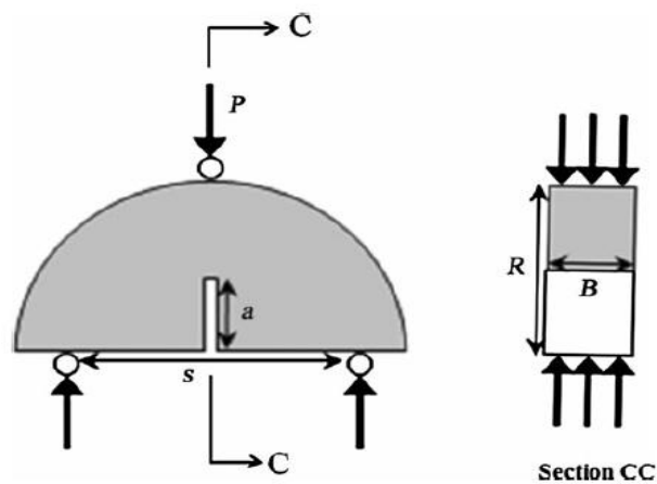
شکل ۲. شرایط بارگذاری [۱۳]
