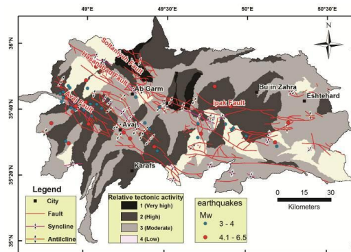
شکل ۱۵. نقشه پراکندگی زمین‌لرزه‌ها بر پهنه‌بندی زمین‌ساخت فعال منطقه
